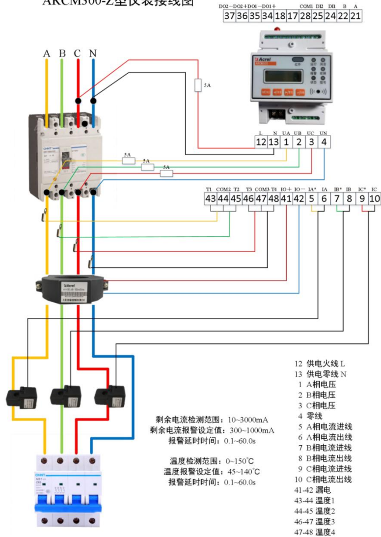
ARCM300-Z型仪表接线图
